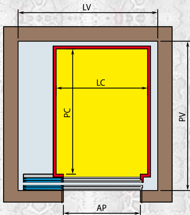
MOD. 1AT2SN/DX UN ACCESSO PORTE TELESCOPICHE DUE ANTE
