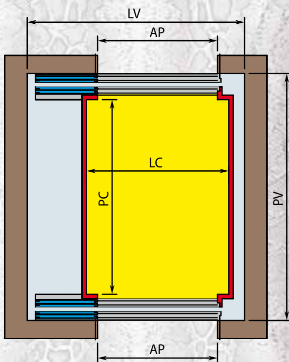
MOD. 2AOT2SN/DX DUE ACCESSI OPPOSTI PORTE TELESCOPICHE DUE ANTE
